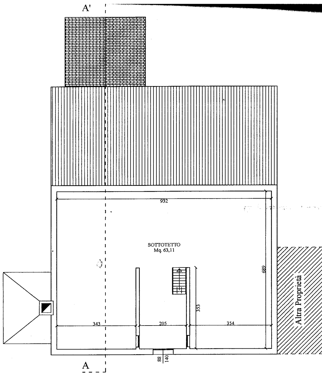
PIANTA SOTTOTETTO
