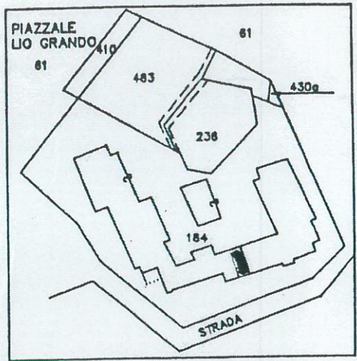
COMUNE DI VENEZIA ESTRATTO MAPPA 1:2000 SEZIONE DI BURANO FOGLIO 36 - MAPP. 184 C.T. - C.E.U.
